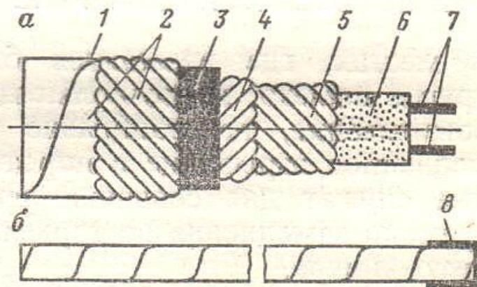
Рис. 18. Детонирующий шнур ДША:
