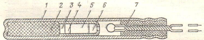
Рис. 13. Схема электродетонаторов короткозамедленного и замедленного действия: 1—гильза; 2—заряд бризантного ВВ; 3—колпачок замедлителя; 4—заряд инициирующего ВВ; 5—замедляющий состав; 6—зажигательный состав; 7—электровоспламенитель
