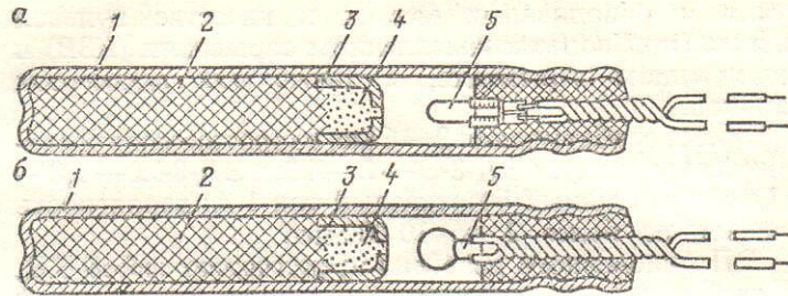
Рис. 12. Схема электродетонатора мгновенного действия: а—ЭД-8-Ж (с жестким закреплением мостика накаливания); б—ЭД-8-Э (с эластично закрепленным мостиком накаливания); 1—гильза; 2—вторичный заряд бризантного ВВ; 3—чашечка; 4—заряд инициирующего ВВ; 5—электровоспламенитель
