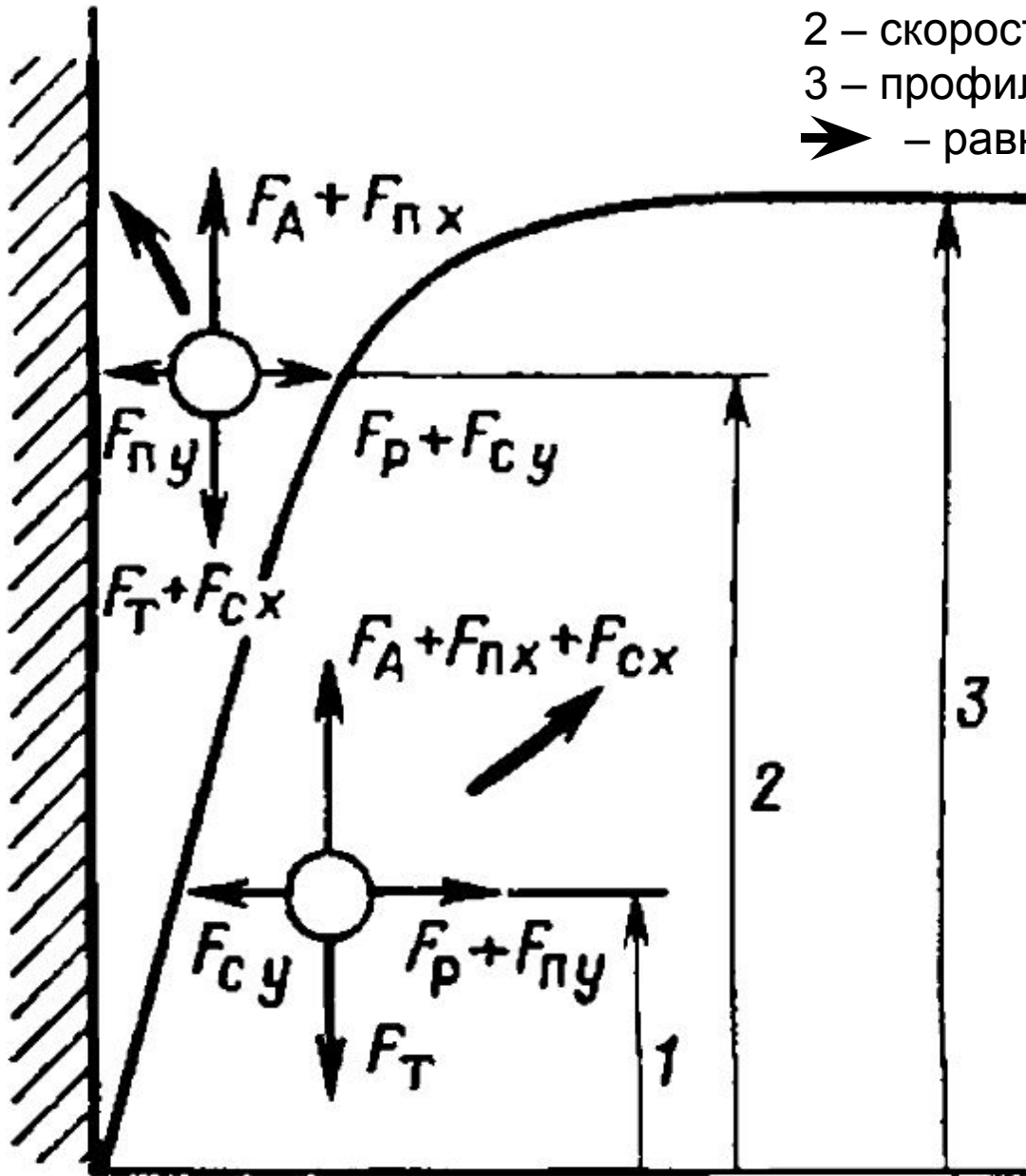
Схема сил, действующих на каплю в потоке пара
