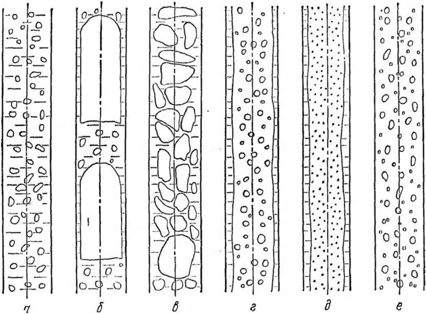
Режимы течения двухфазного потока в вертикальной трубе: а – пузырьковый; б – снарядный; в – эмульсионный; г – дисперсно-кольцевой; д – кольцевой; е – дисперсный.
