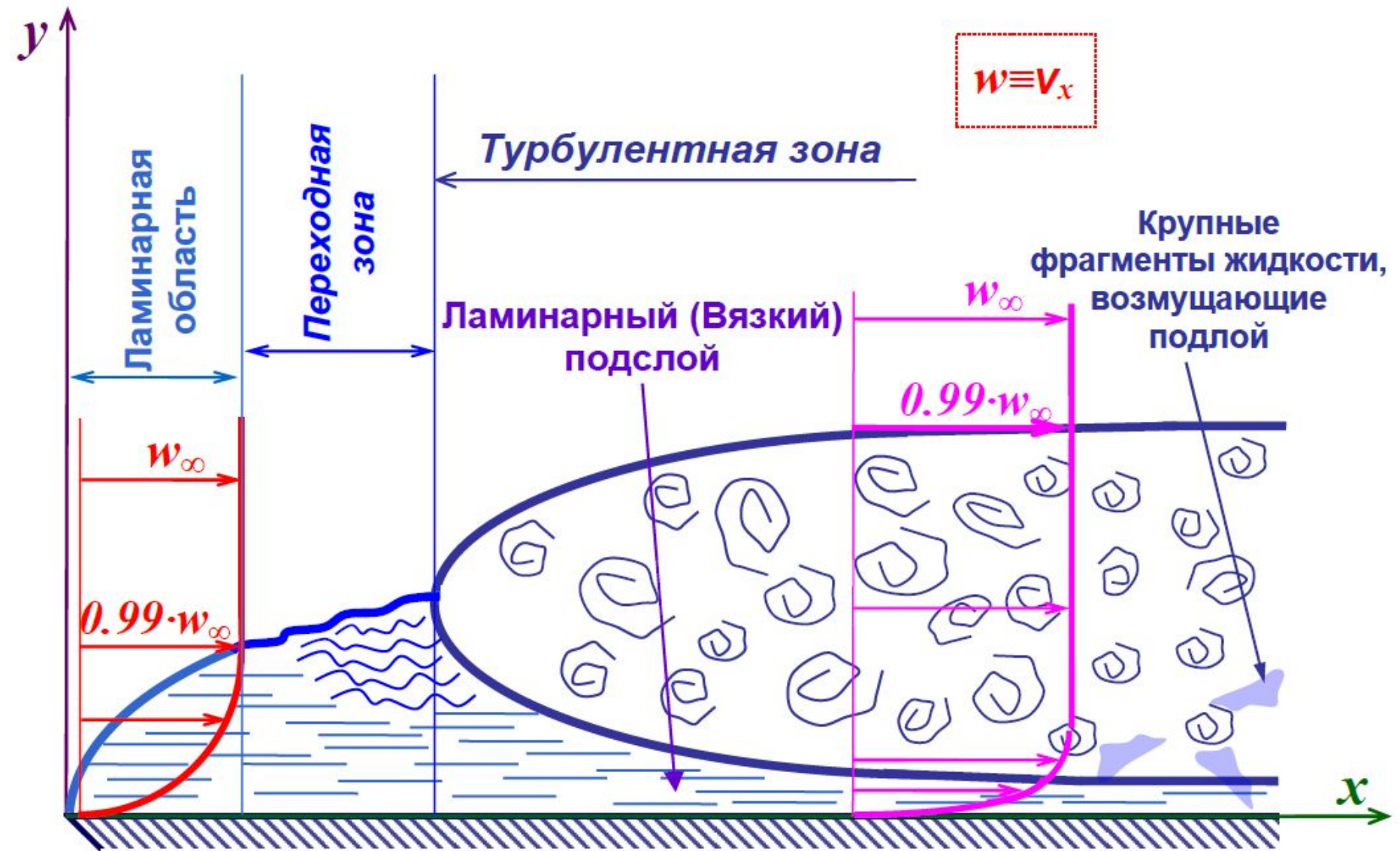
Развитие плоского гидродинамического пограничного слоя
