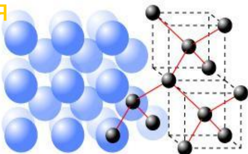
УПАКОВКА АТОМОВ И ПРОСТРАНСТВЕННАЯ РЕШЕТКА АЛМАЗА
