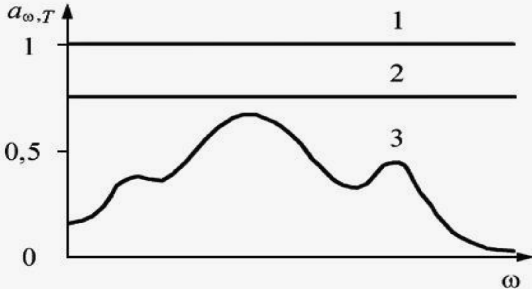
Рис. 2. Спектральная поглотительная способность тела: 1 – абсолютно черное тело; 2 – серое тело; 3 – реальное тело
