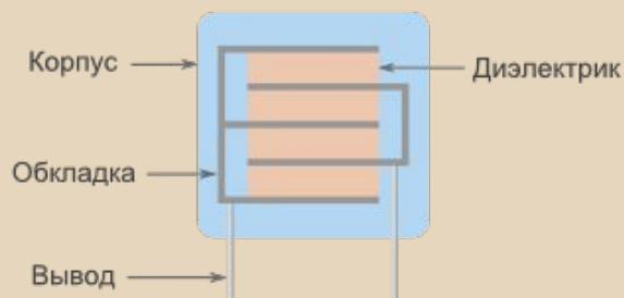
Радиальные пленочные конденсаторы
