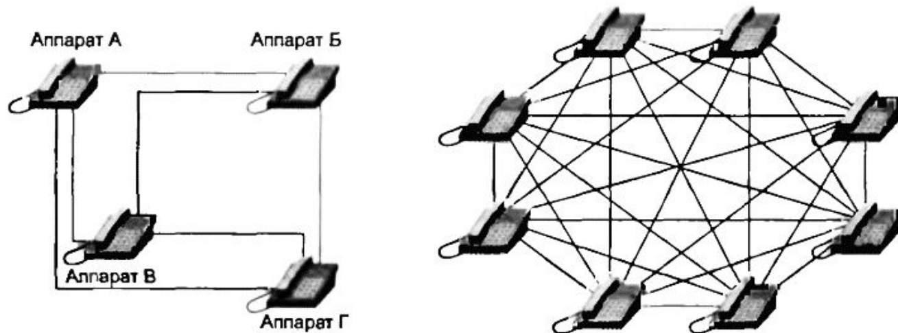
Схема без использования телефонной станции (коммутатора)
