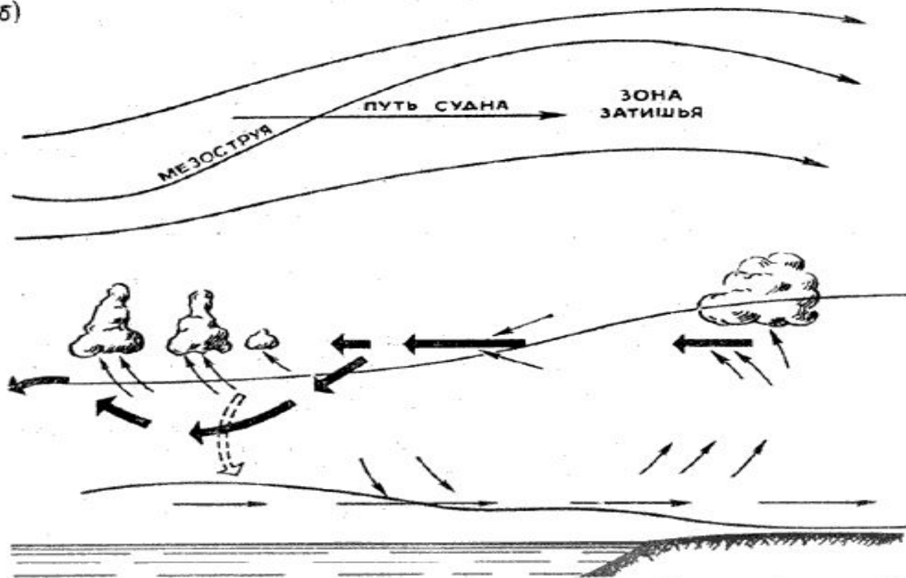
Схема бризовой циркуляции.
