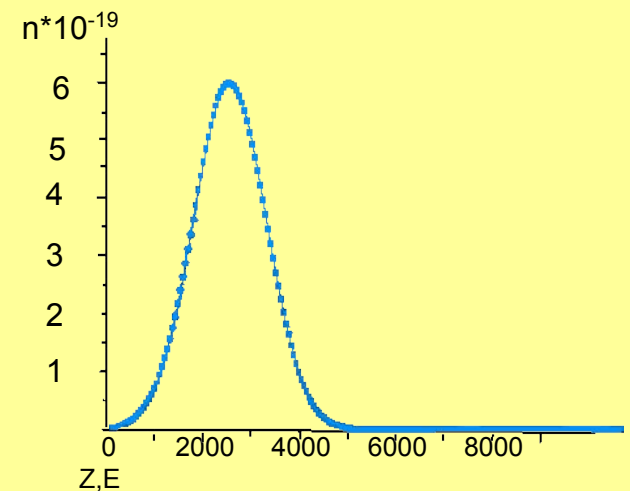
Распределение имплантированных ионов фосфора в кристалле кремния, полученное с помощью программного пакета SRIM-2003
