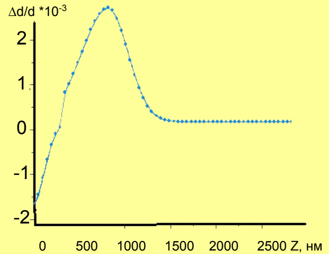
Профиль деформации в приповерхностных слоях кристалла, имплантированного ионами фосфора
