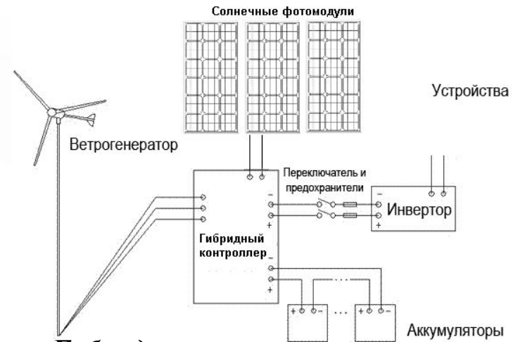
Гибридная автономная система – солнце-ветер
