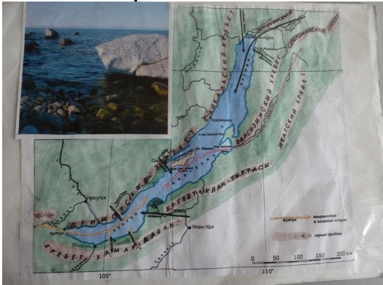
Основные ветра на Байкале
