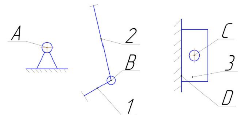
Кинематические пары
