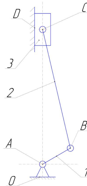
Кинематические звенья
