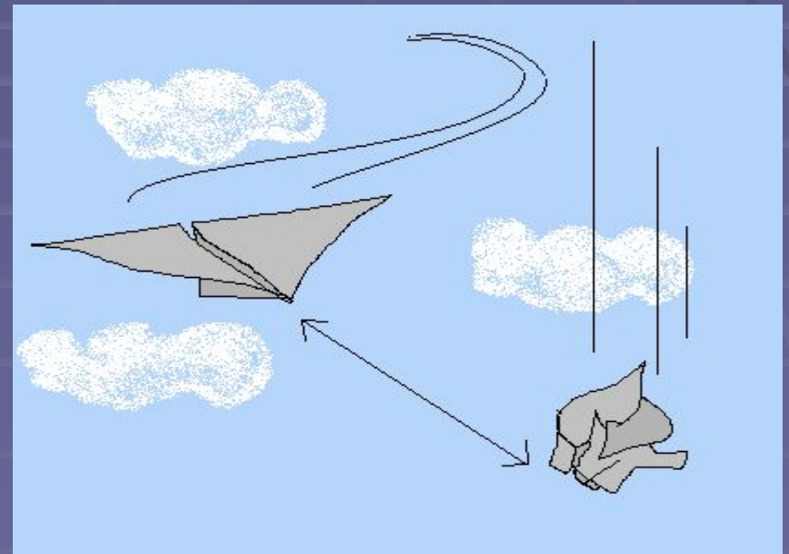
Сила сопротивления воздуха останавливает самолётик
