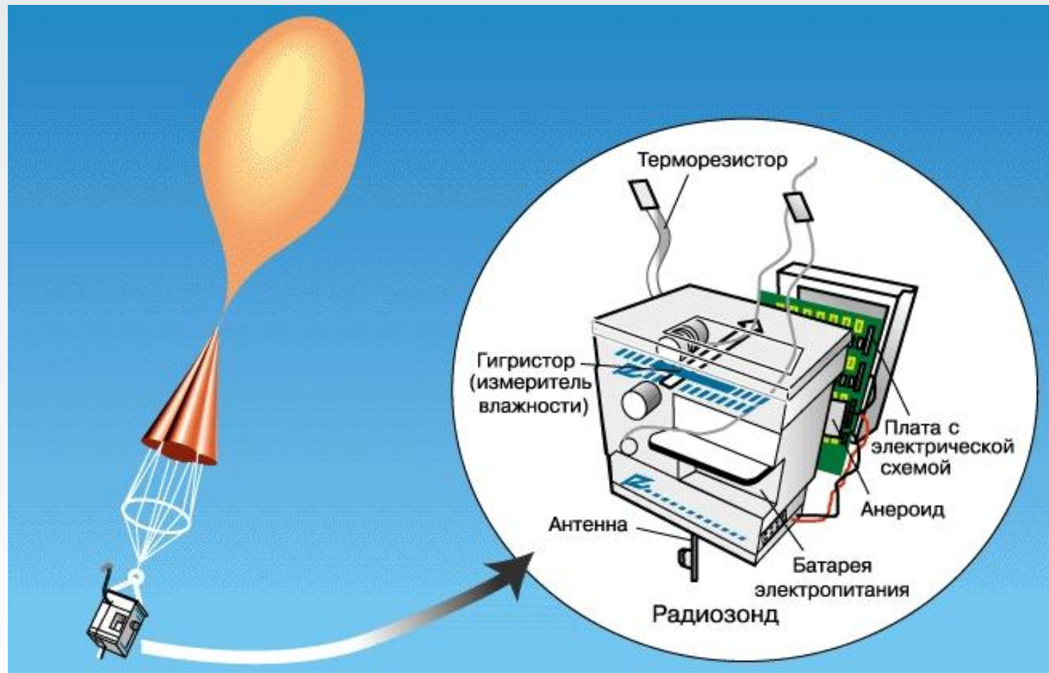
Рис. 1.2.3. Радиозонд.
