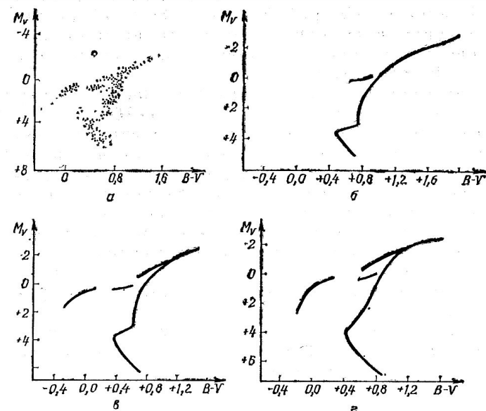
Диаграмма цвет — светимость: a — для шарового скопления М 3 (кружочком отмечена цефеида); b — для шаровых скоплений 47 Тукана, М 71 и М 69, богатых тяжелыми элементами; c — для шаровых скоплений М 3, М 72 и М 5 со средним содержанием тяжелых элементов; d — для шаровых скоплений М 13 и М 80, \omega Кентавра и NGC 6752, бедных тяжелыми элементами
