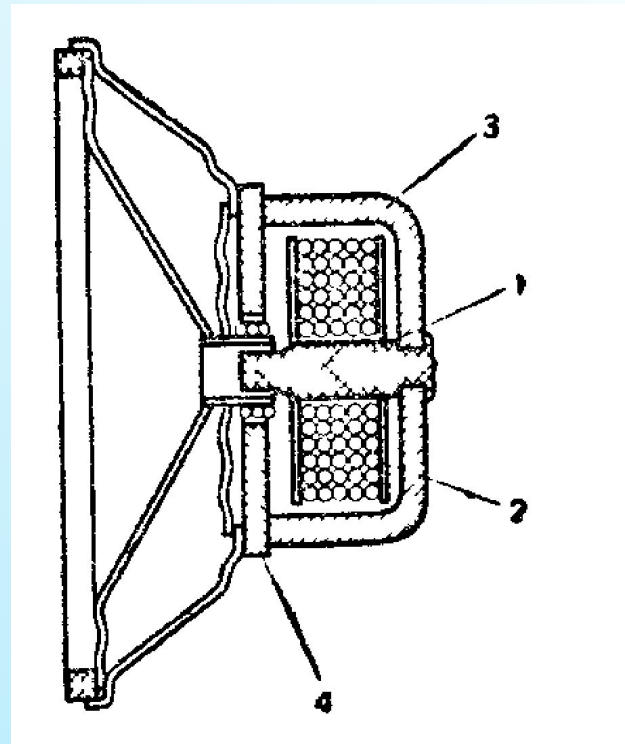
Рис. 8. Устройство громкоговорителя с подмагничиванием.
