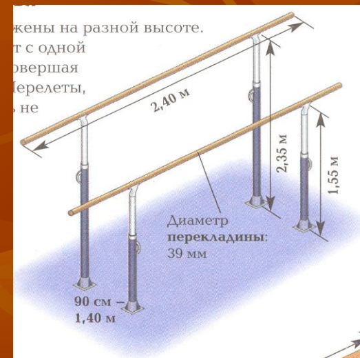
Брусья разной высоты
