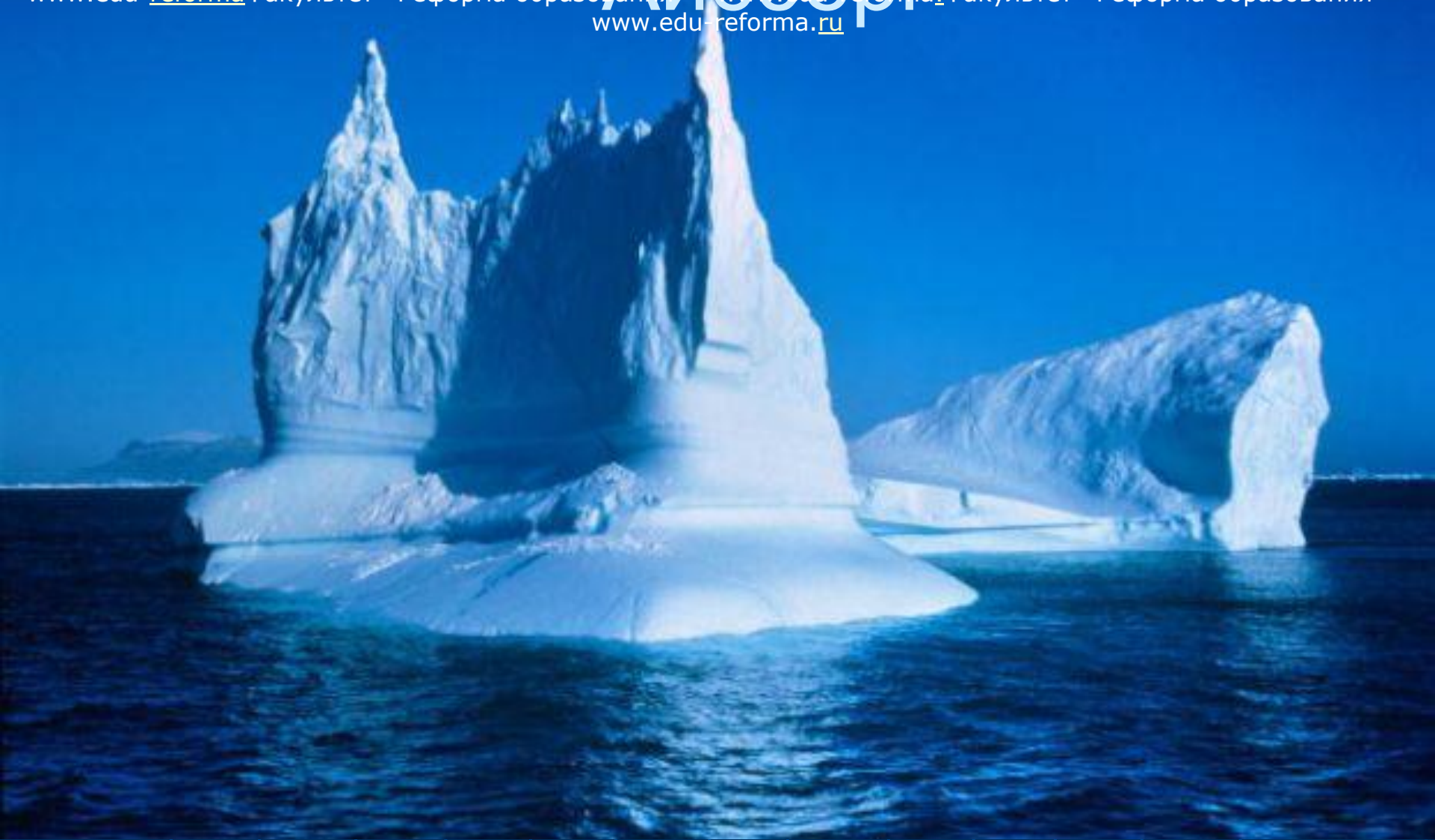
Льды Арктики имеют толщину до 4 км. Материковые льды сползают в океан и образуют айсберги – плавающие ледяные глыбы.
