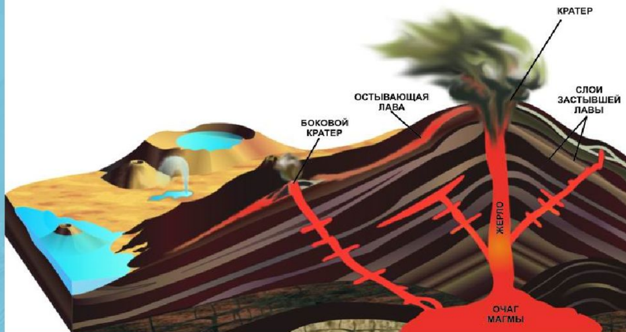
Строение вулкана.
