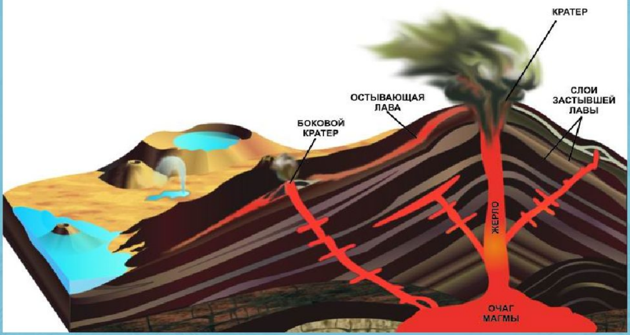
Строение вулкана.
