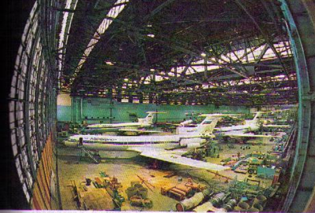
3. Сборка самолетов Ту-154М на авиазаводе в г. Самаре
