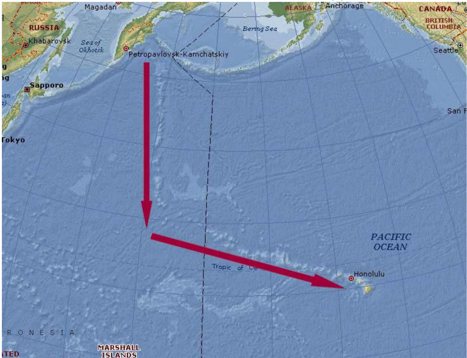
След на Тихоокеанской плите от Гавайского восходящего потока
