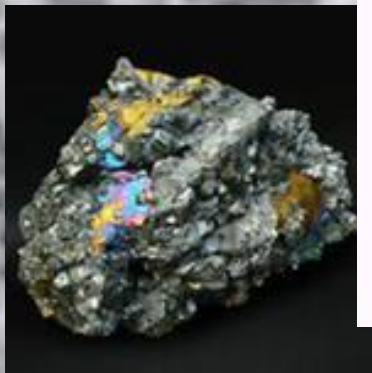
Халькопирит – медная руда
