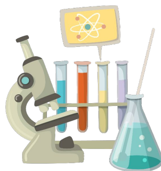
химия
