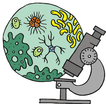
биология
