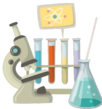
химия
