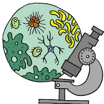
биология
