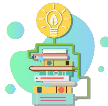
физика
