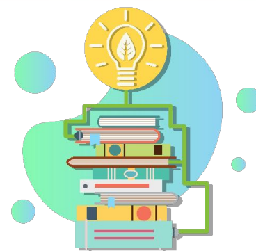
физика
