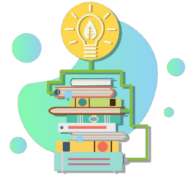
физика
