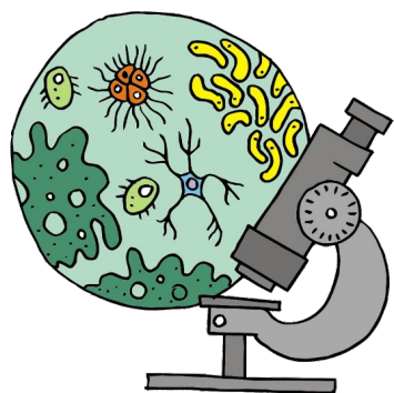
биология
