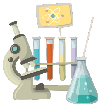
химия
