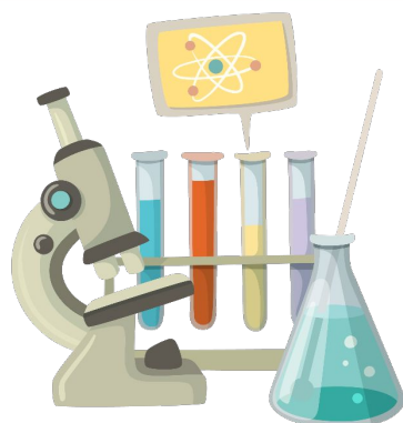
химия
