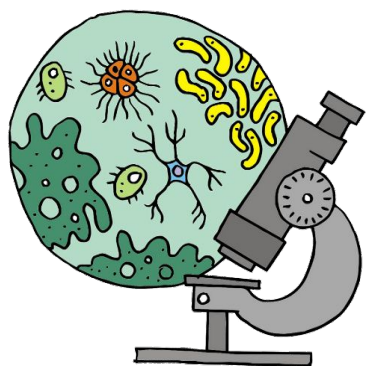
биология
