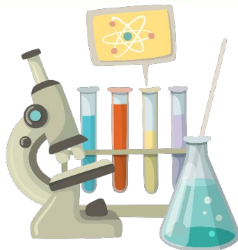
химия
