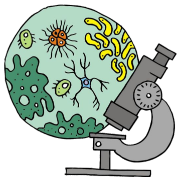
биология
