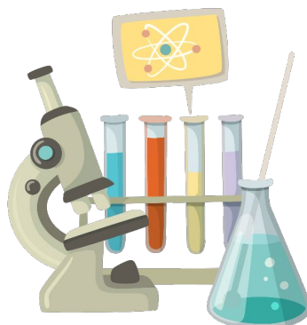
химия
