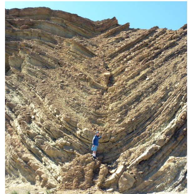
синклиальная складка
