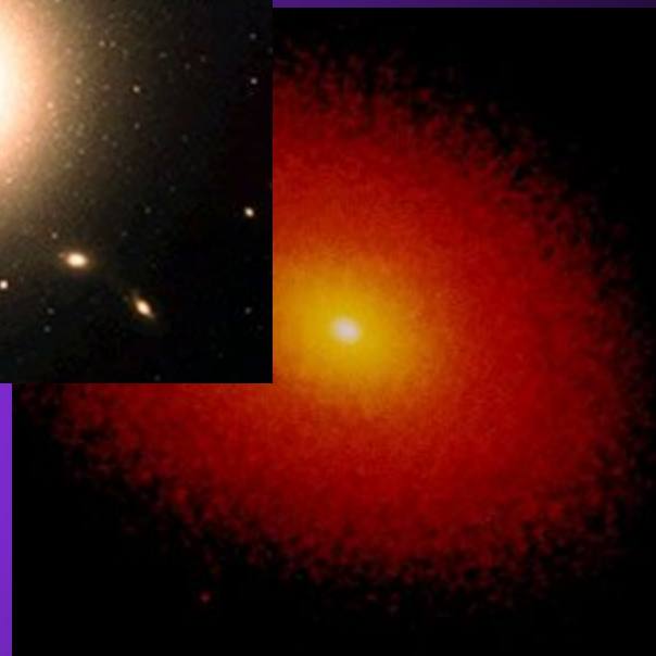
Эллиптические галактики
