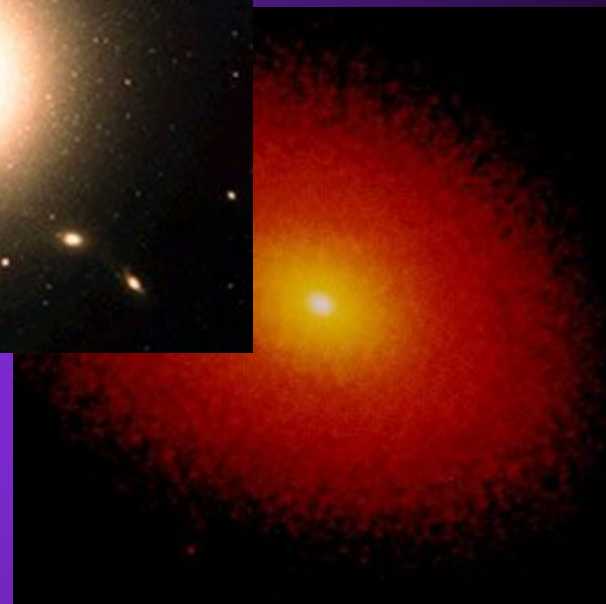
Эллиптические галактики
