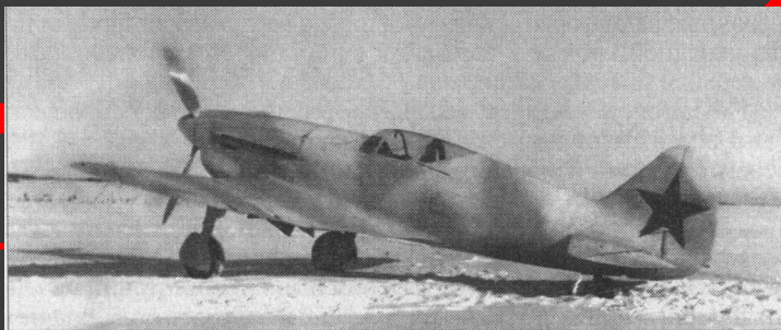
Истребитель тяжелый пушечный ИТП (М-1) Н.Н. Поликарпова с мотором М-107
