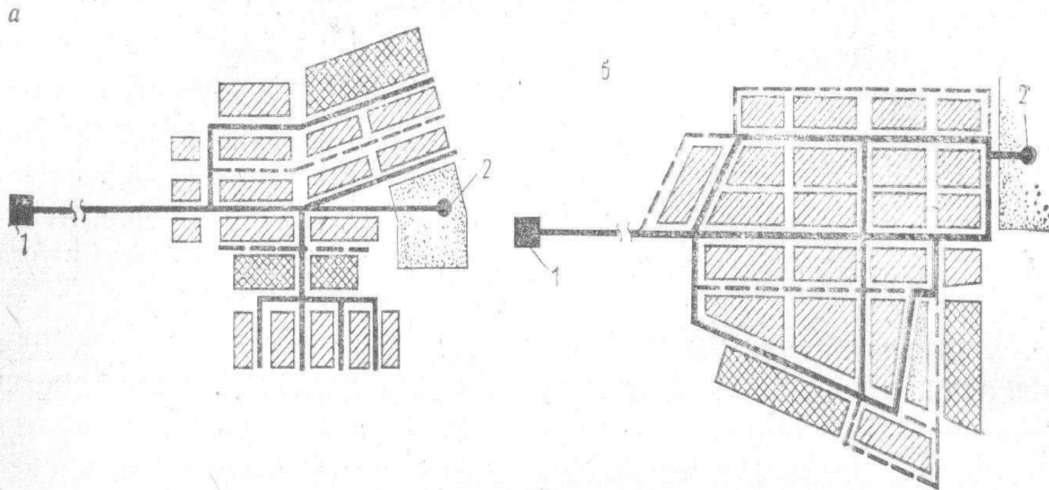
Рис. 51. Водопроводная сеть
