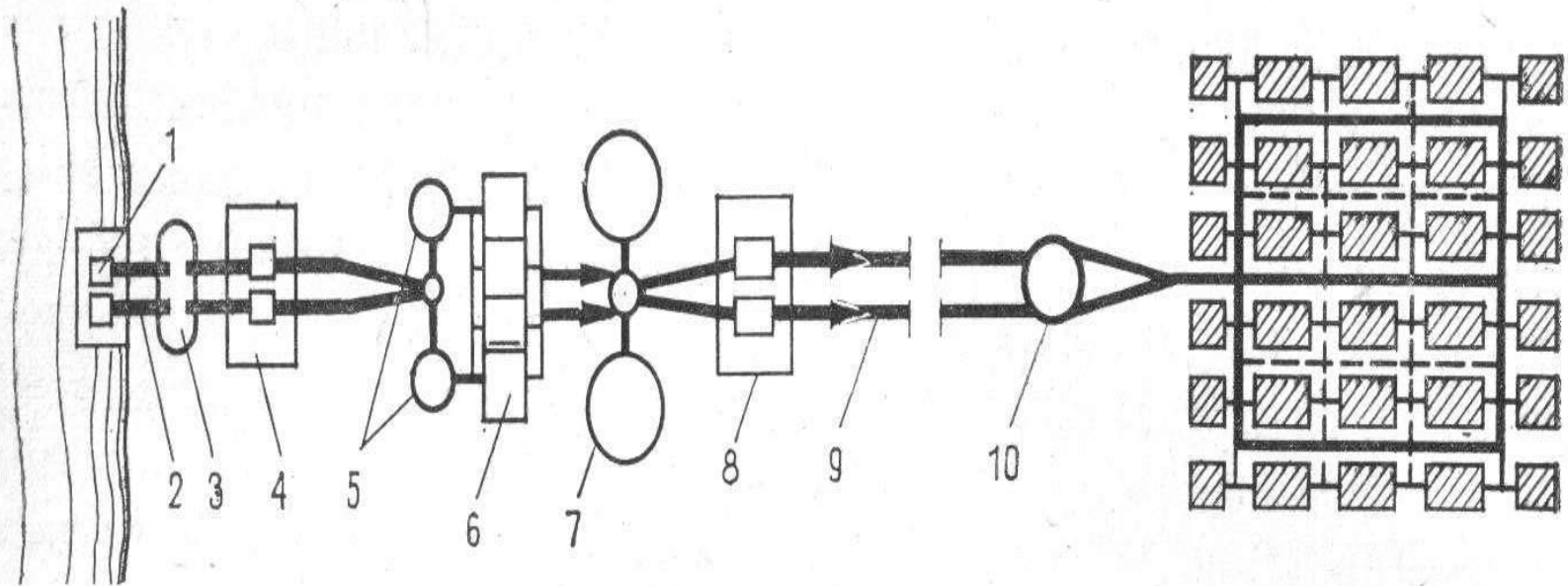
Рис. 50. Схема водоснабжения города
