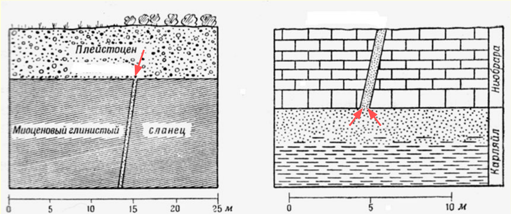
Дайка нептуническая
