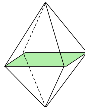
Тетрагональная дипирамида
