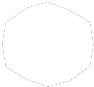
Сечение - дигексагон
