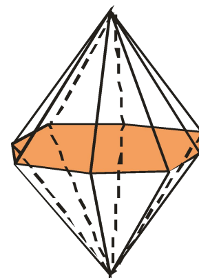
Дитетрагональная дипирамида
