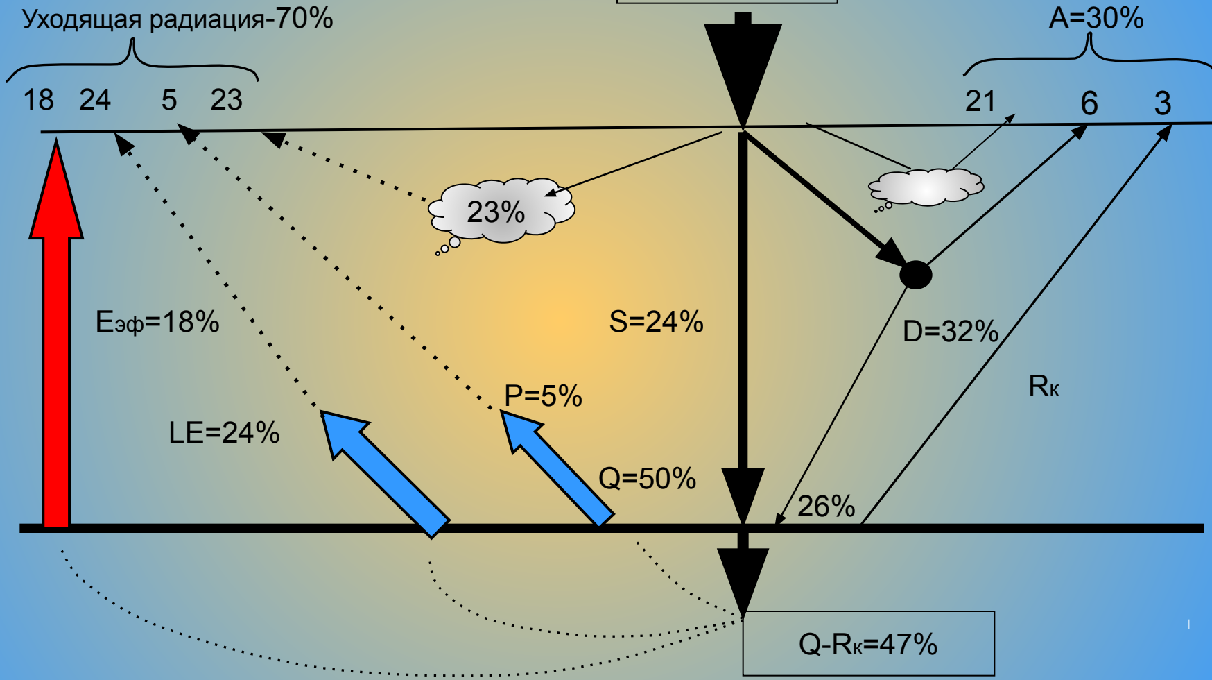
Рис.1 Схема радиационного и теплового балансов земной поверхности
