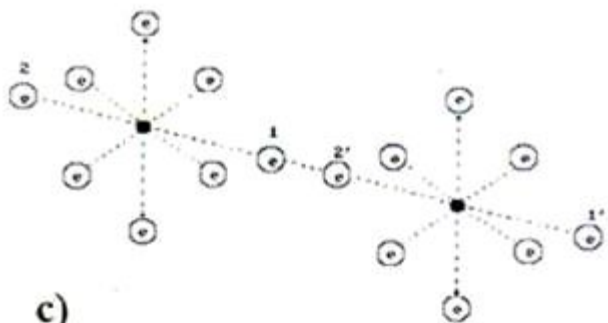
Молекула кислорода
