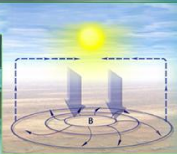
АНТИЦИКЛОН
