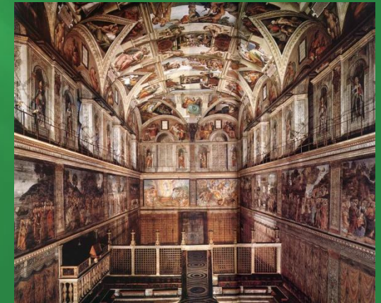
Сикстинская капелла
