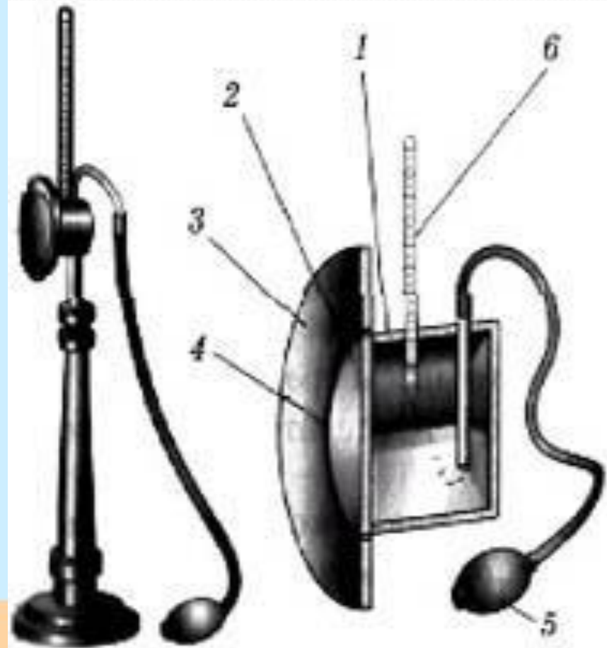
Гигрометр конденсационный
