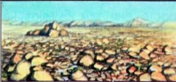
Каменистая пустыня
