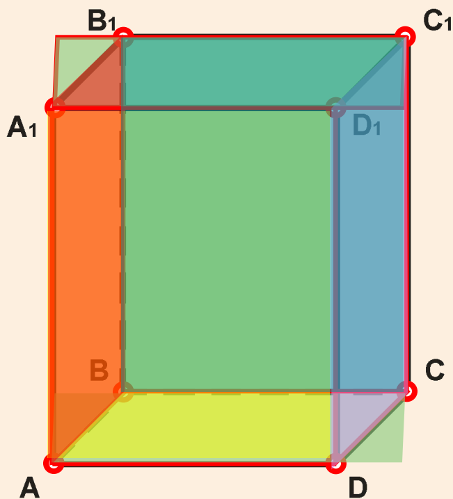
Параллелепипед
