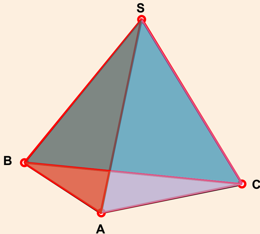
Тетраэдр
