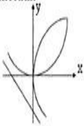
Декартов лист
