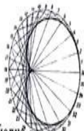
кардиоиды
