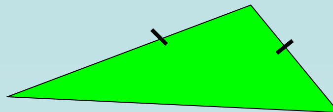
Произвольный треугольник
