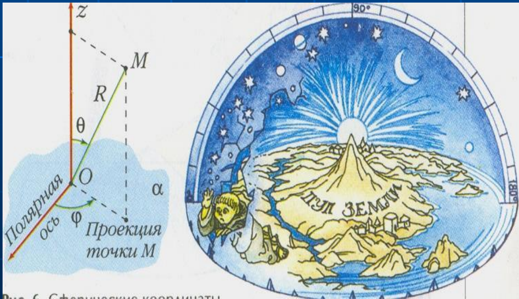
Рис. 6. Сферические координаты.
