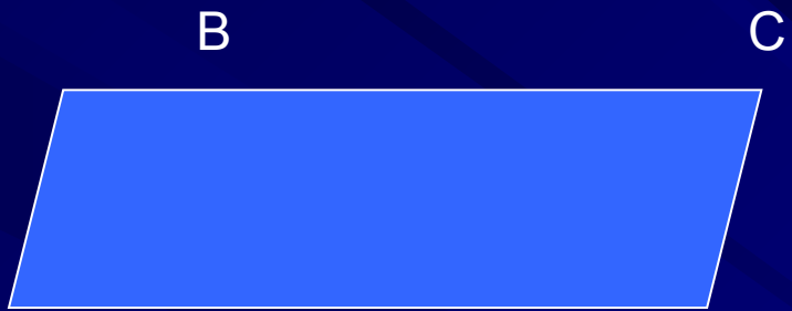
параллелограмм
