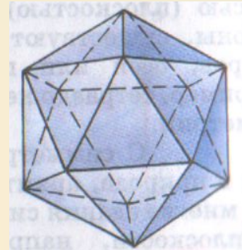
Икосаэдр
