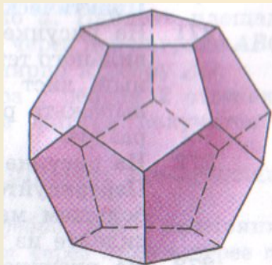
Додекаэдр
