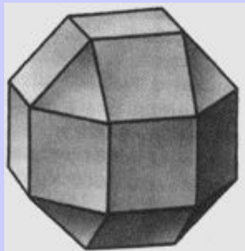
ромбокубооктаэдр
