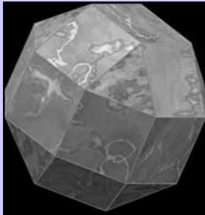
Псевдоромбокубооктаэдр
