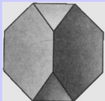
Усеченный тетраэдр
