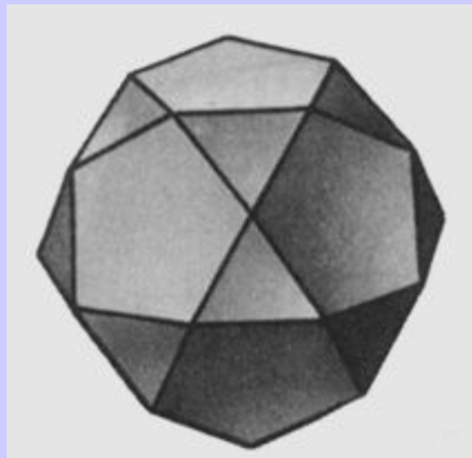
кубооктаэдр
