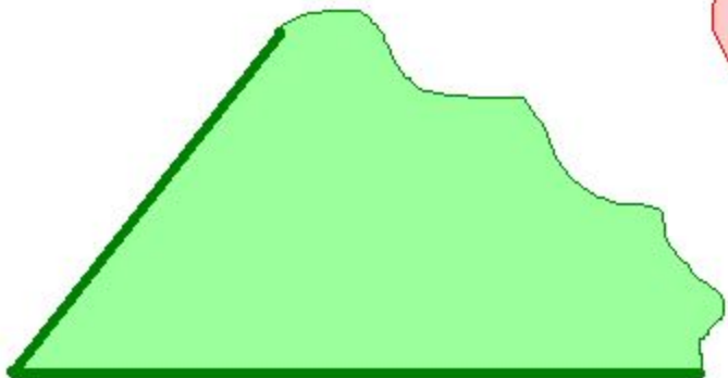
Острый угол
