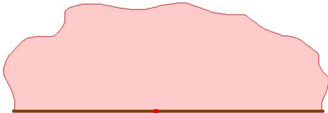
Развернутый угол
