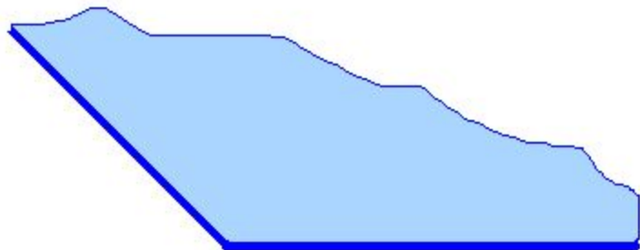
Тупой угол
