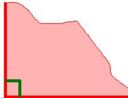
Прямой угол
