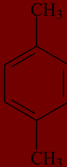
п-ксилол (1,4-диметилбензол)
