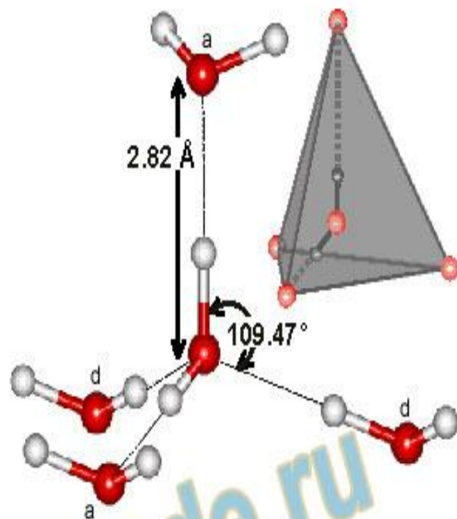
Рис. Тетраэдрическая структура воды
