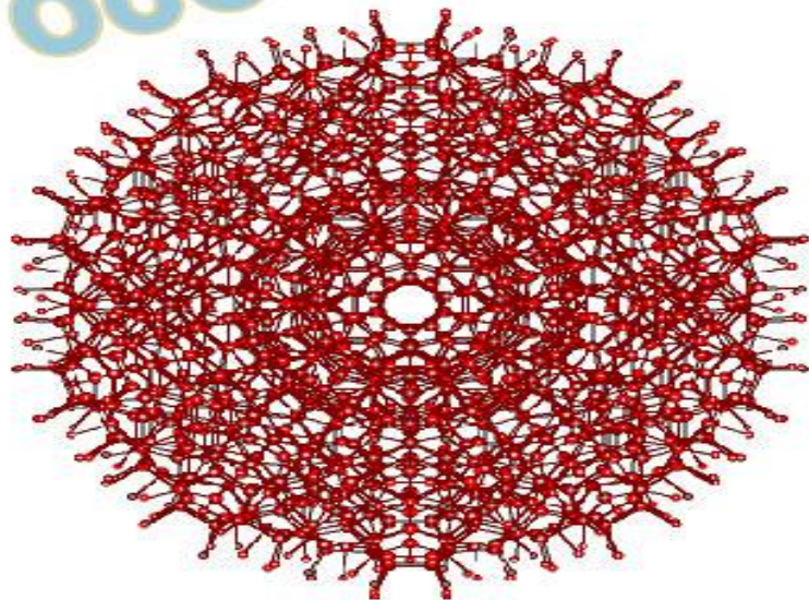
Рис. Гигантский икосаэдр воды
