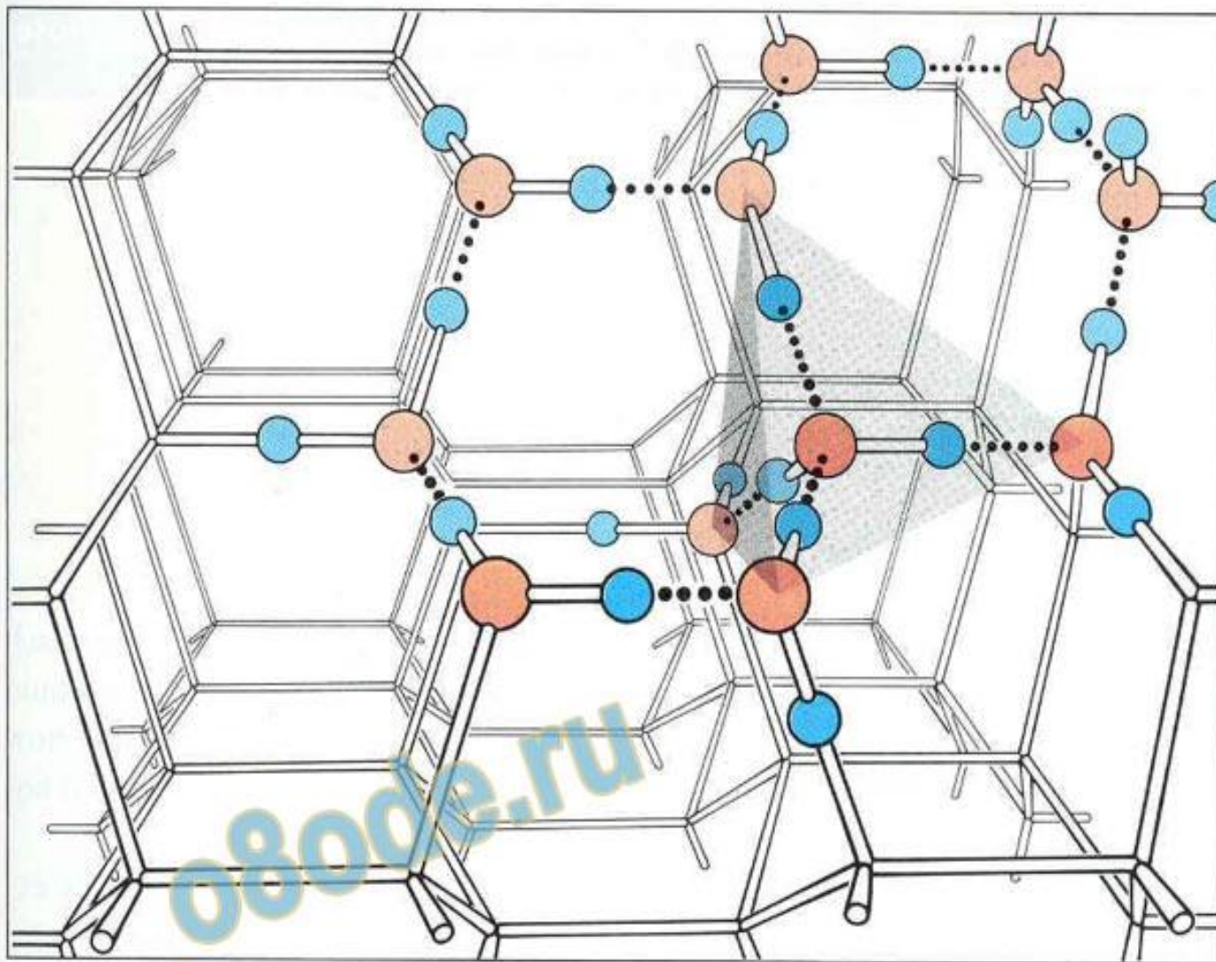
Рис. Кристаллическая структура льда
