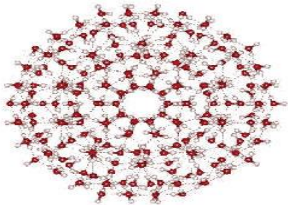
Рис. Формирование икосаэдра воды
