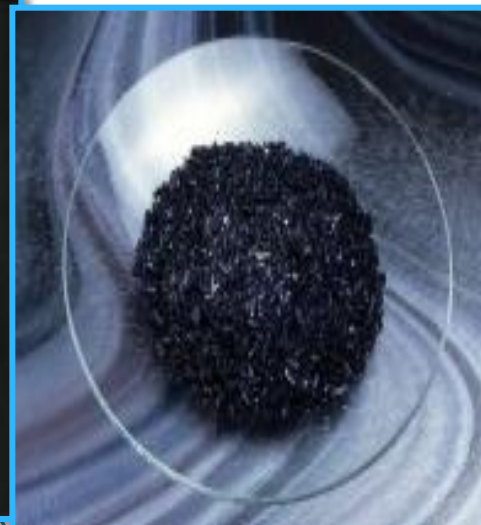
\text{KMnO}_4
