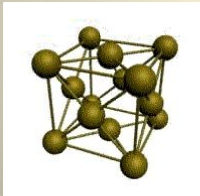
Гранецентрированная
