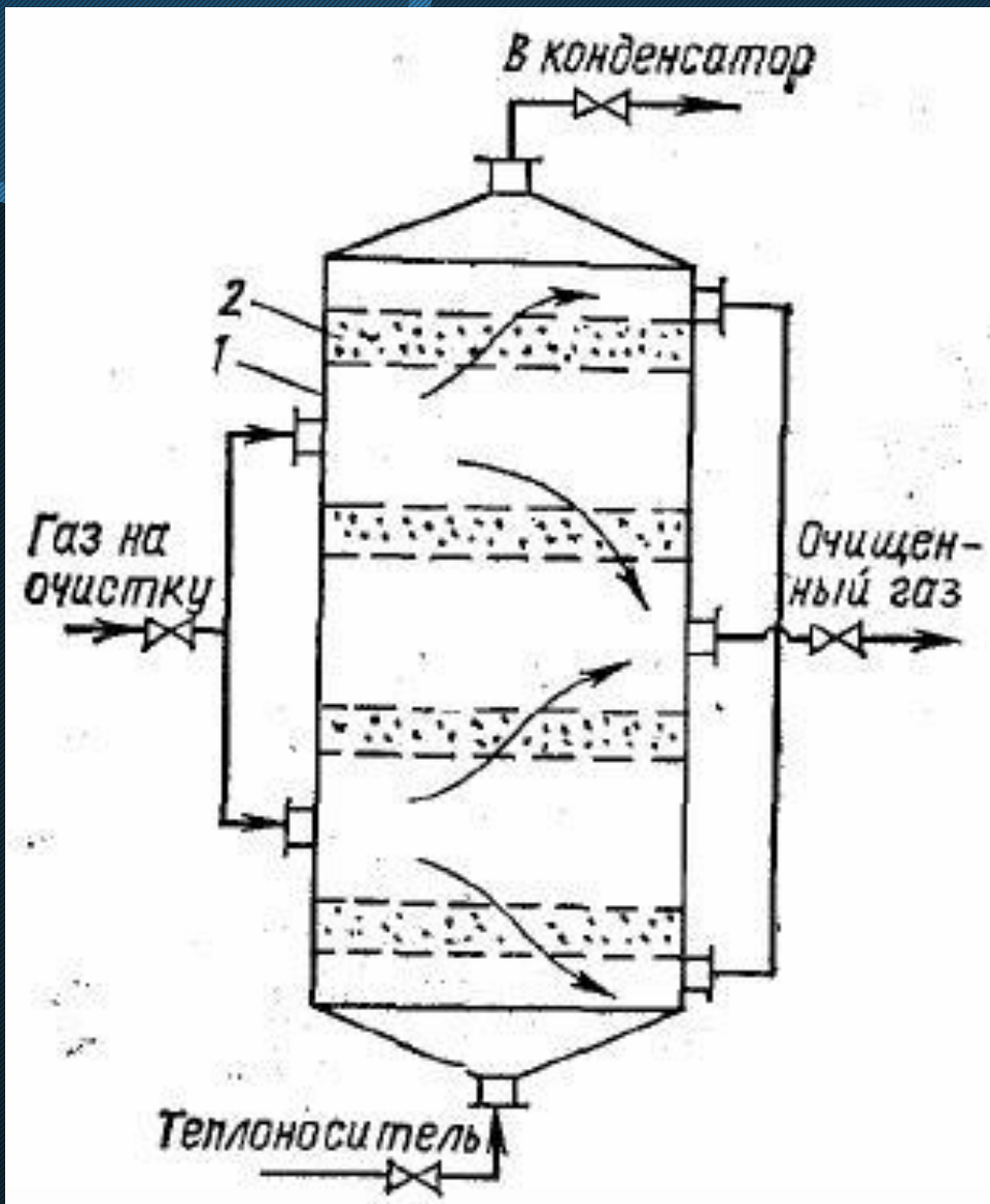
Рис. 1. Адсорбер полочного типа с неподвижными слоями адсорбента
